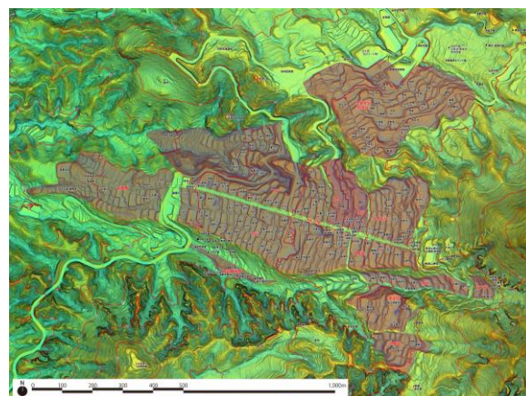
図表 48 英彦山全体レーザー測量図
