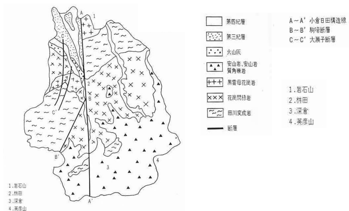
図表 15 地質図
